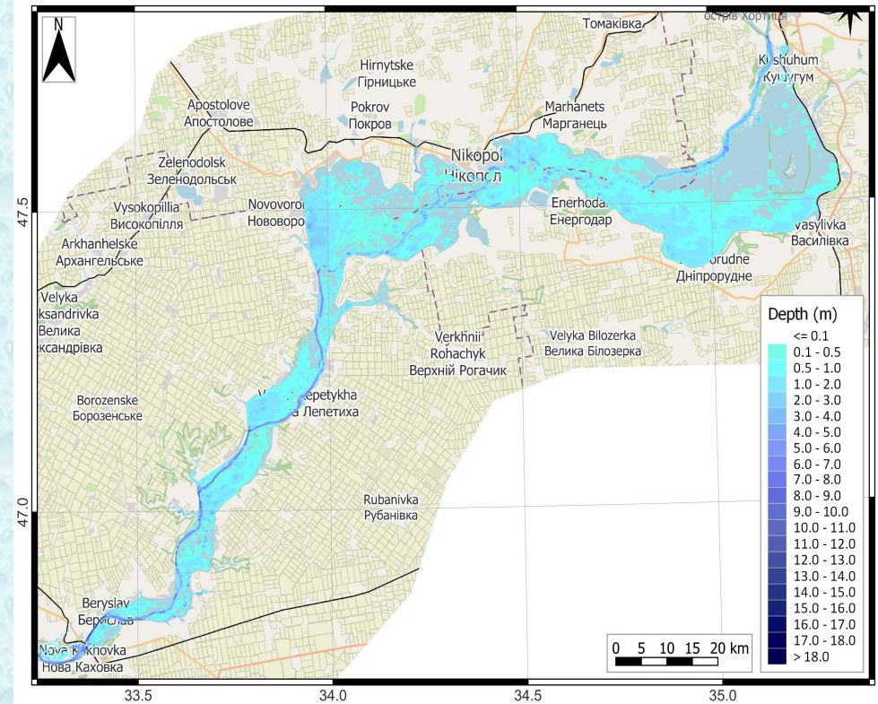
Розподіли глибин у Каховському водосховищі: початковий, перед проривом греблі ГЕС при рівні Каховського водосховища 15 м БС і кінцевий після прориву греблі. (15.06.2023)
