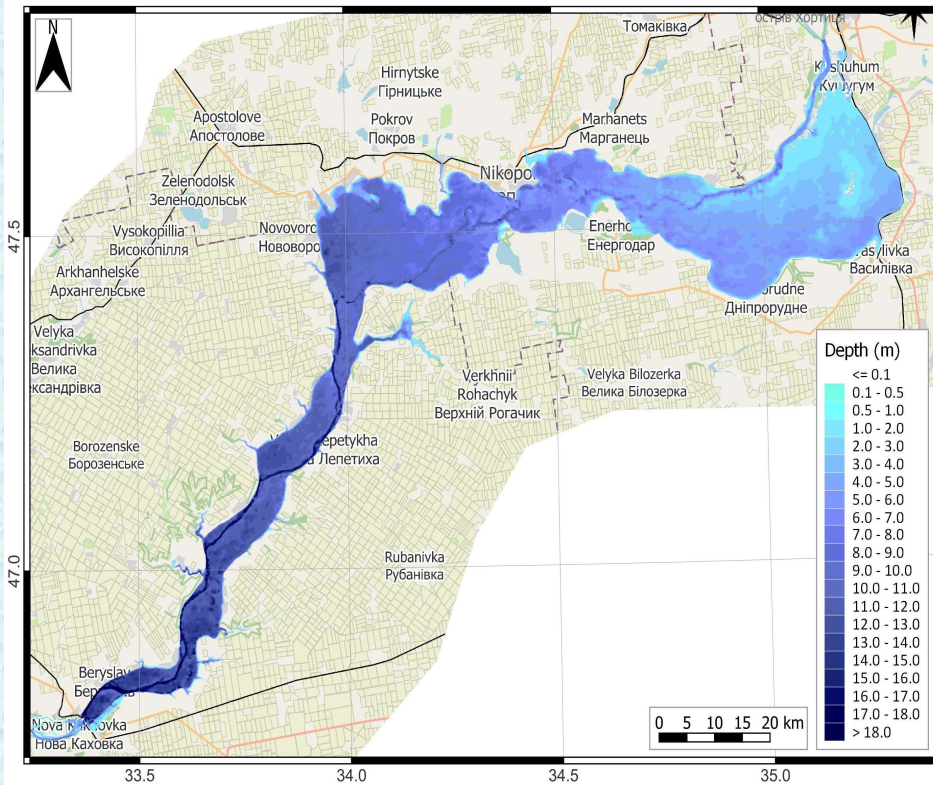
Розподіли глибин у Каховському водосховищі: початковий, перед проривом греблі ГЕС при рівні Каховського водосховища 15 м БС і кінцевий після прориву греблі. (15.06.2023)
